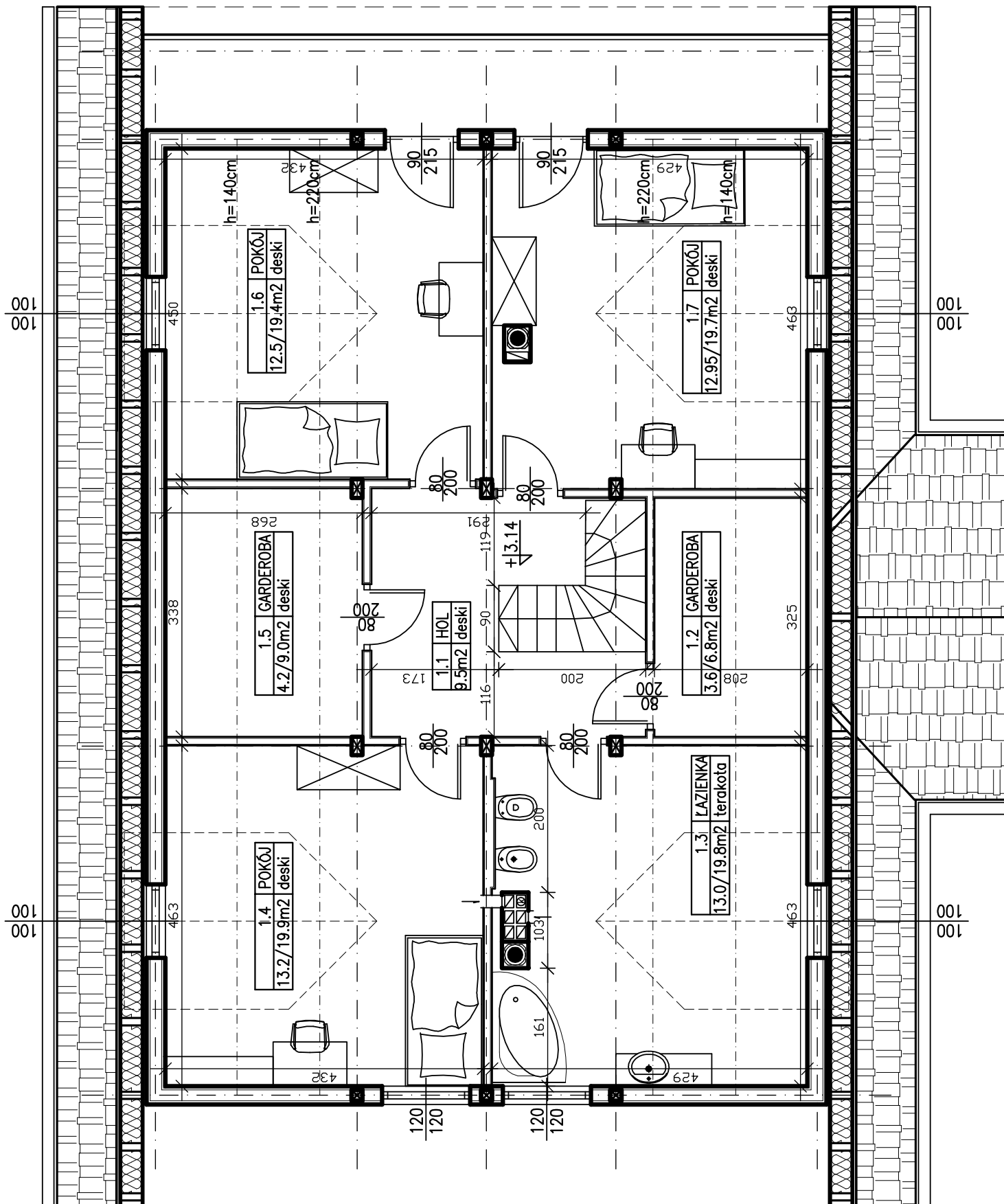
RZUT PODDASZA SKALA 1:100
